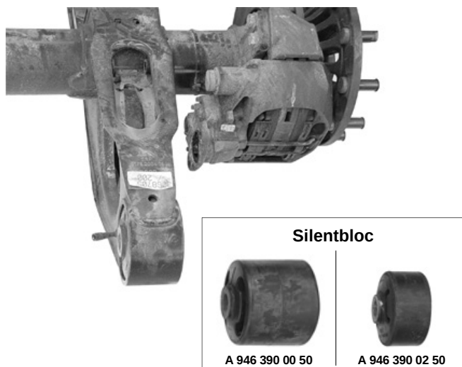
Fig. 2 : Extraire le silentbloc.
