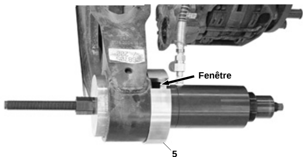
Fig. 7 : Le silentbloc est rétracté.
