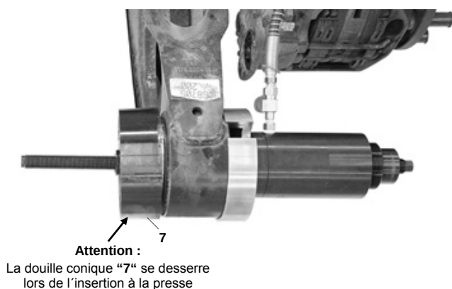
Fig. 7 : Le silentbloc est rétracté.
