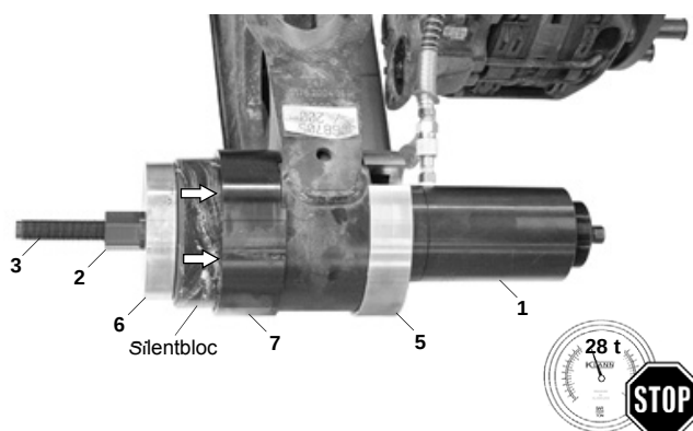
Fig. 6 : La douille conique se desserre pendant l'insertion à la presse.
