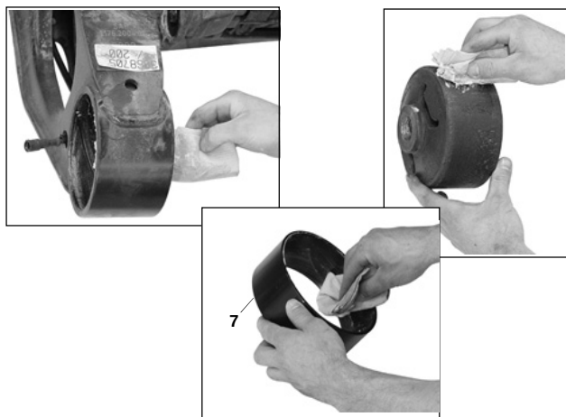
Fig. 4 : Graisser l'alésage du silentbloc, le silentbloc et la douille conique avec la pâte de montage appropriée.
