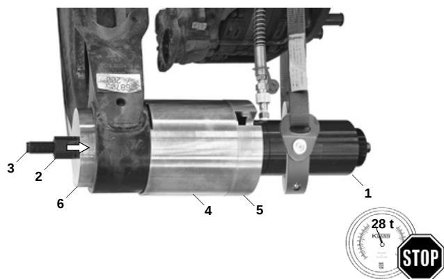
Fig. 3 : Le silentbloc est retiré.
