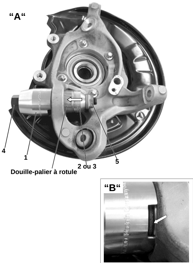
Fig.4 Pose de la douille-palier à rotule
