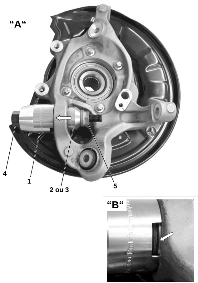
Fig.4 Pose de la douille-palier à rotule
